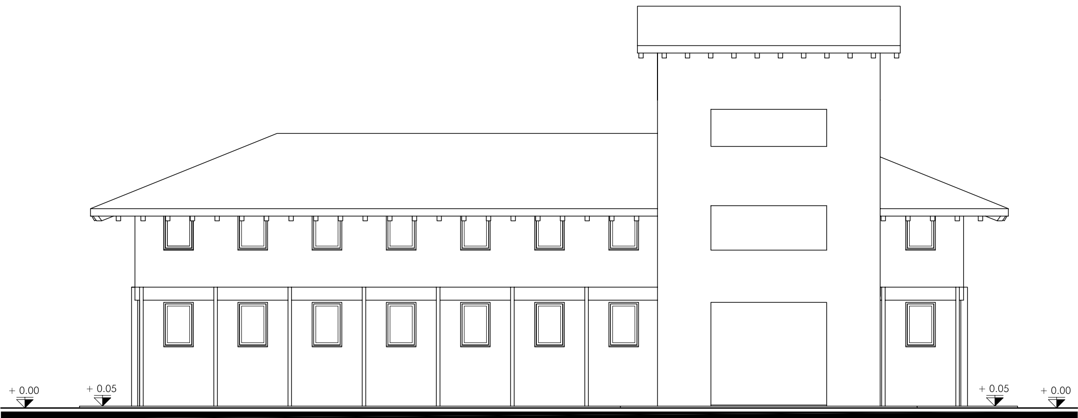
PROSPETTO OVEST
